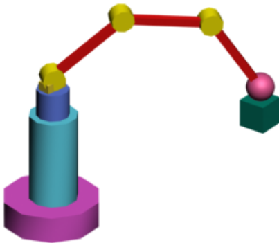
IK structure
